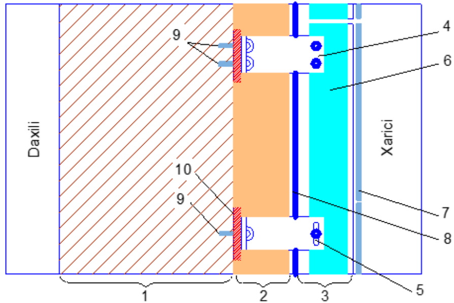
Şəkil 2. Hava aralaylı asma fasad sistemlərinin prinsipial konstruktiv sxemi (şaquli kəsik):
