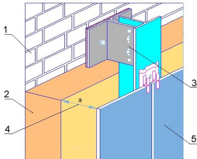
Şəkil 1. Hava aralaylı asma fasad sisteminin prinsipial konstruktiv sxemi (fəza şəkli): 1-əsas (divar); 2-istilik izolyasiya qatı; 3-yükdaşıyan karkas elementləri; 4-hava aralayı; 5-ekran
