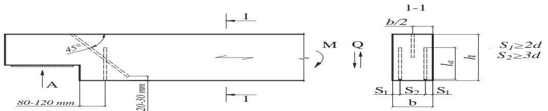
Şəkil 19. Tirin dayağında kəsmənin gücləndirilməsi
