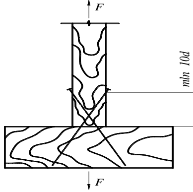
Şəkil 13. Mismarların çəpinə vurulması
