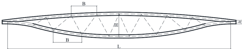
Şəkil 22. Linzaşəkilli fermaların sxemi
