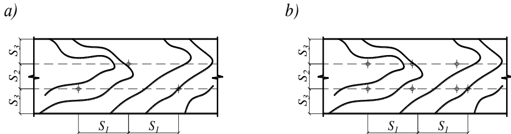
a — şahmatvari düzülüş; b — ikicərgəli düzülüş Şəkil 17. Daxilə yapışdırılmış polad nagellərlə birləşmələr
