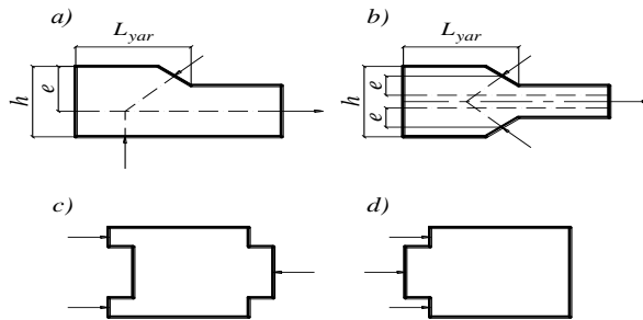
a – qeyri-simmetrik; b – simmetrik; c, d – birləşmələrdə yarıma sxemləri Şəkil 5. Birləşmə elementlərində oyuqlar
