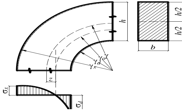
Şəkil 25. Əyilib yapışdırılan çərçivələrin əyrixətli hissəsində gərginliyin təyin olunmasının hesablama sxemi
