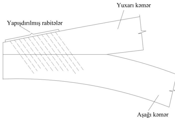
Şəkil 23. Linzaşəkilli fermanın dayaq düyününün sxemi
