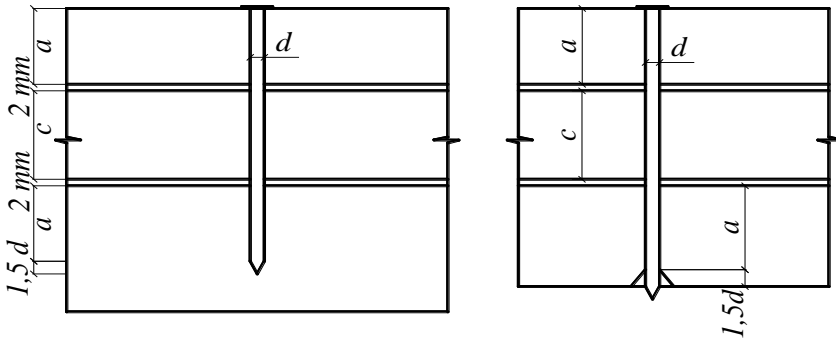
Şəkil 11. Mismarın ucunun sancılmasının hesablama uzunluğunun təyini
