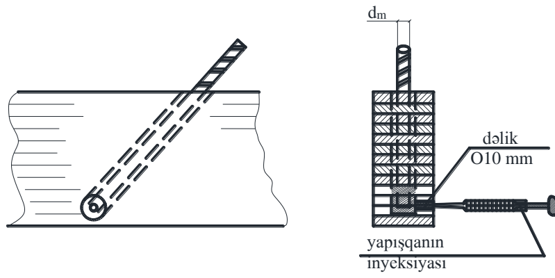
Şəkil 31. Təzyiq altında yapışqanın verilməsi sxemi
