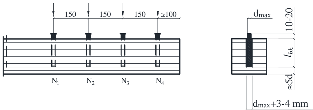
Şəkil 32. Təcrübə üçün sınaq nümunələrinin sxemi
