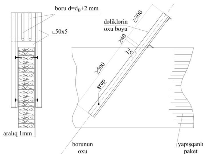
Şəkil 30. Qoyma elementlərin qaynağı və maili dəliklərin deşilməsi üçün şablonun konstruktiv sxemi
