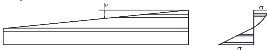
Şəkil 20. Biryamaçlı tir
