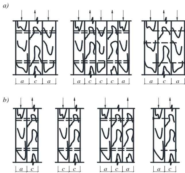
Şəkil 8. Nagel birləşmələri
