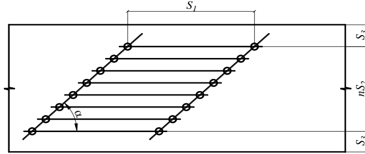
Şəkil 12. Mismarların çəp cərgələrlə yerləşdirilməsi
