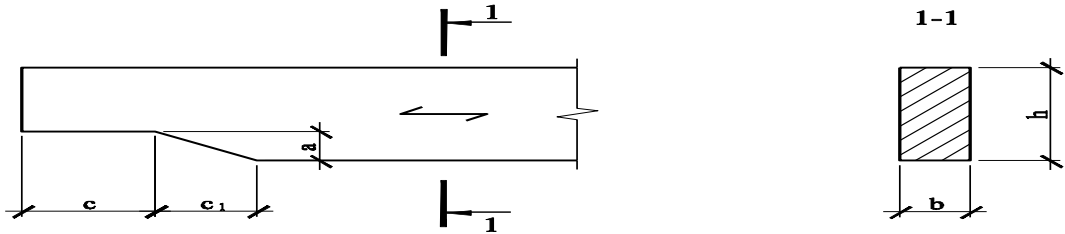
Şəkil 18 . Tirin dayağının biçimli kəsilməsi
