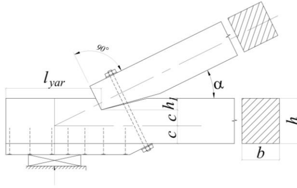
Şəkil 7. Birdiqli alin yarma
