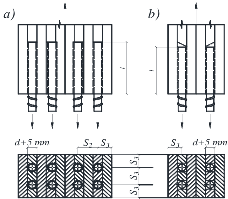
Şəkil 16. Liflər istiqamətində yapışdırılmış dövrü profilli armaturlardan olan içliklərdə birləşmələr
