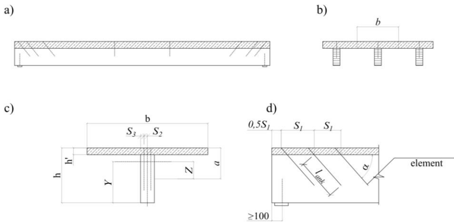
a – ümumi görünüşü; b – en kəsik; c – en kəsiyin həndəsi xarakteristikaları; d – tirin dayaq hissəsi
