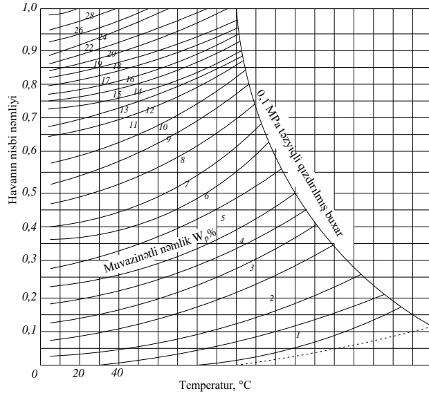
Şəkil 26. Ağacın müvazinətli nəmlik diaqramı
